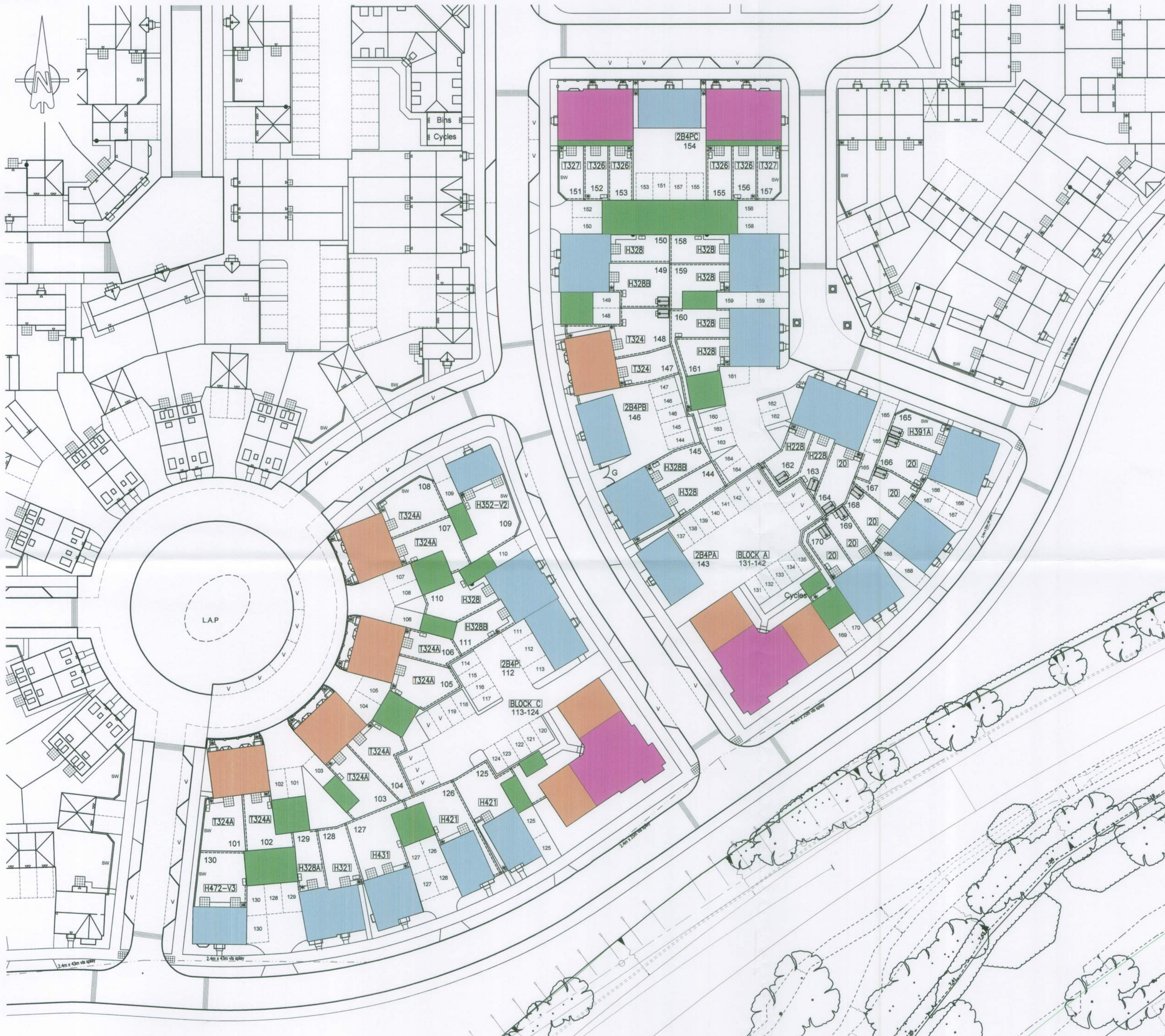
SITE LAYOUT 1:500
