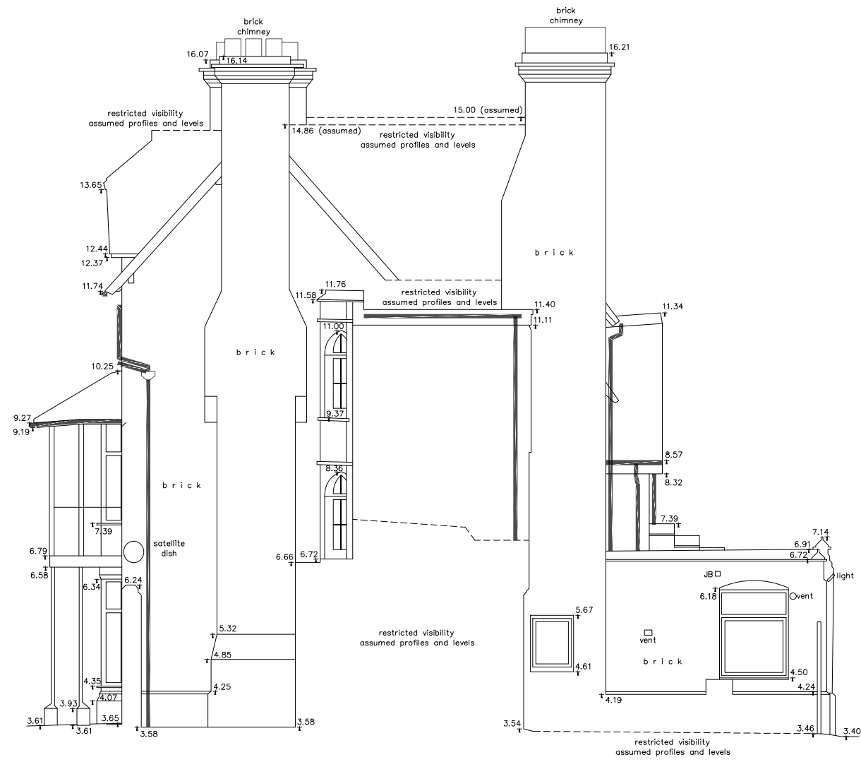
ELEVATION B
