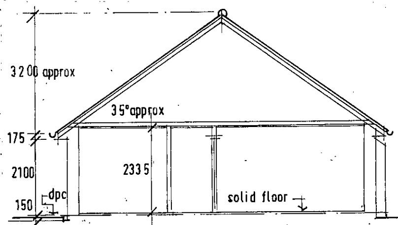
SECTION A-A 1/100
