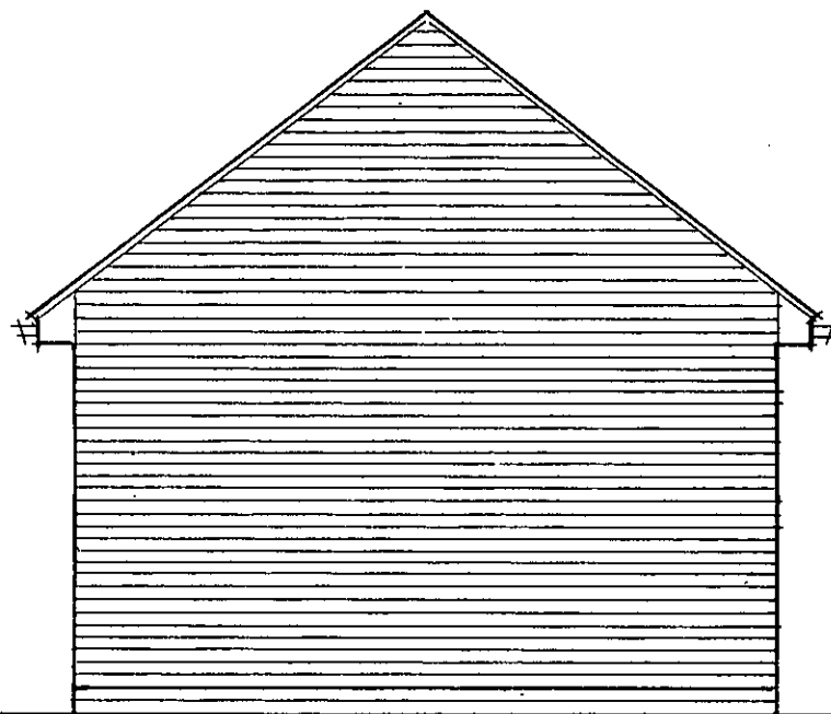
S.E. ELEVATION
