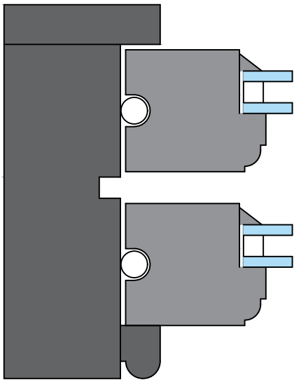
Jamb thru section
