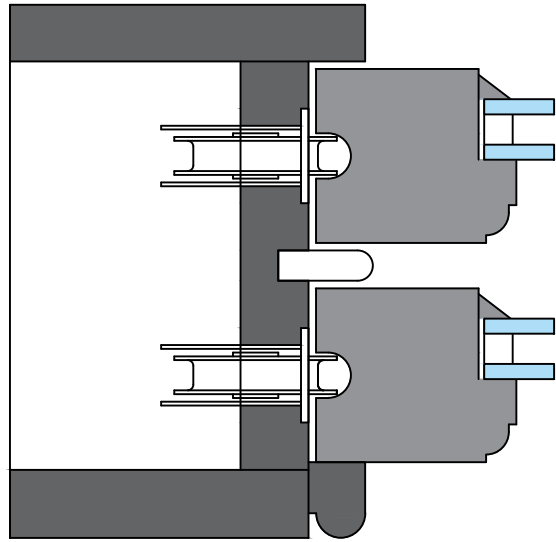
Jamb thru section
