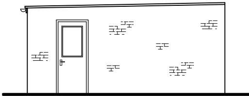
East Elev 1:100 @ A3
