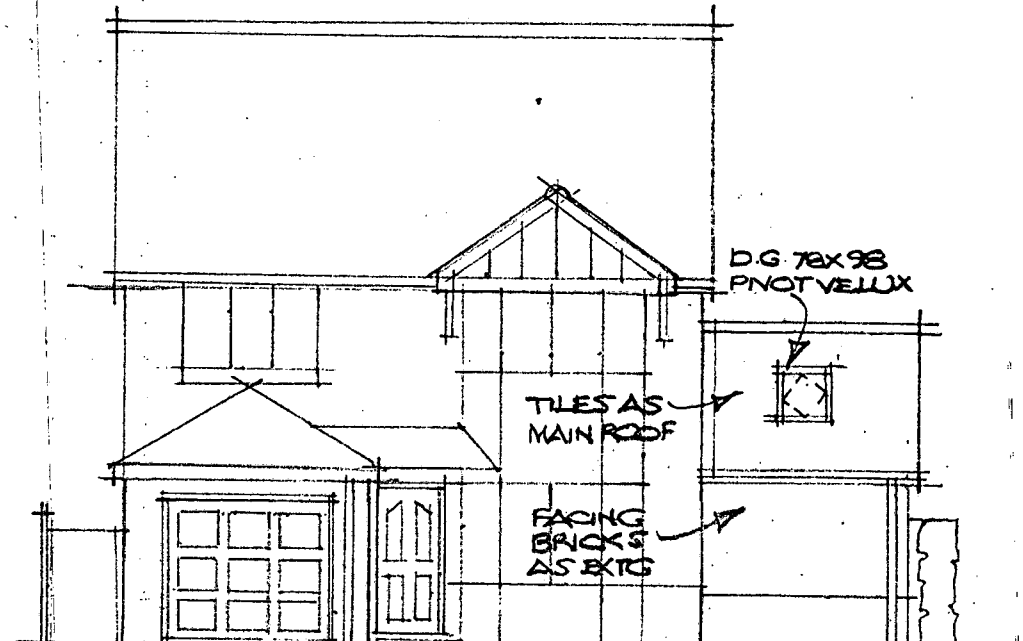
FRONT (S.E.) ELE.
