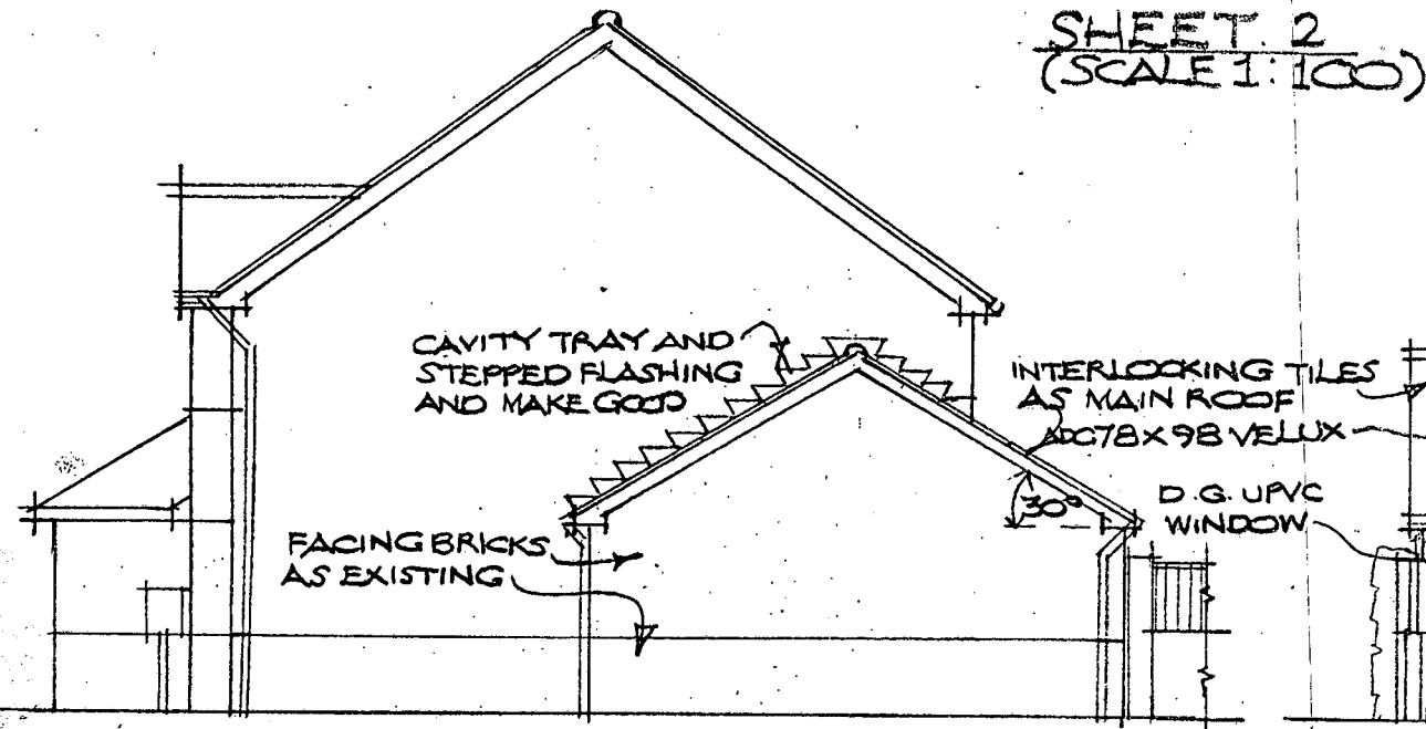
SIDE (N.E.) ELE.
