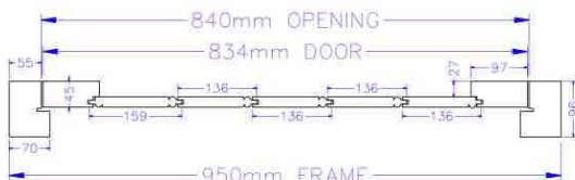
DOOR PLAN SECTION BOTTOM
