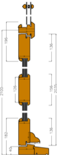
Section V2 (scale 1:4)
