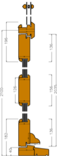
Section V1 (scale 1:4)
