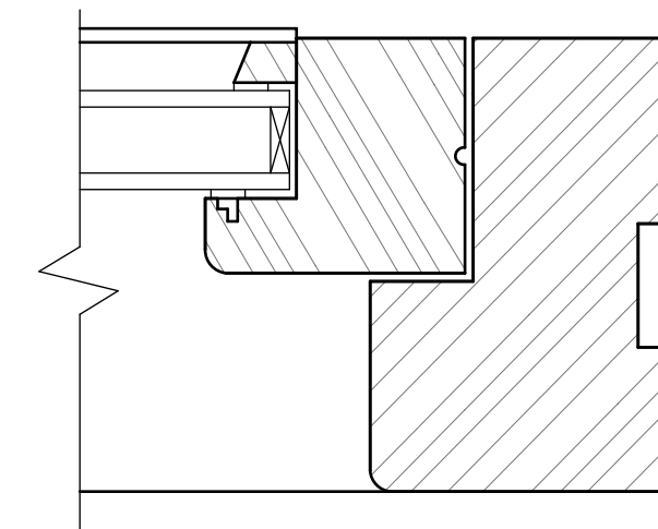
Jamb
