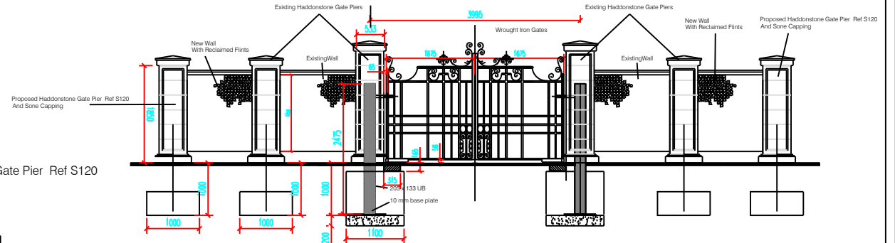
Elevation A
