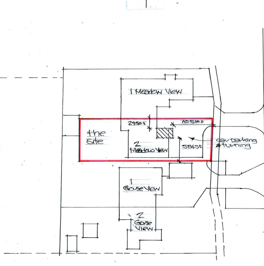
Site Plan 1/500
