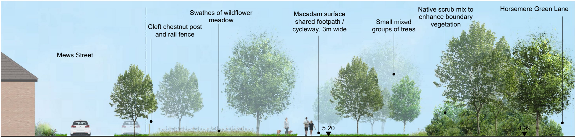
Section 1:200 @ A3
