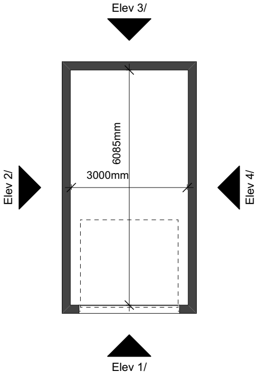
01 Floor Plan Scale: 1:100
