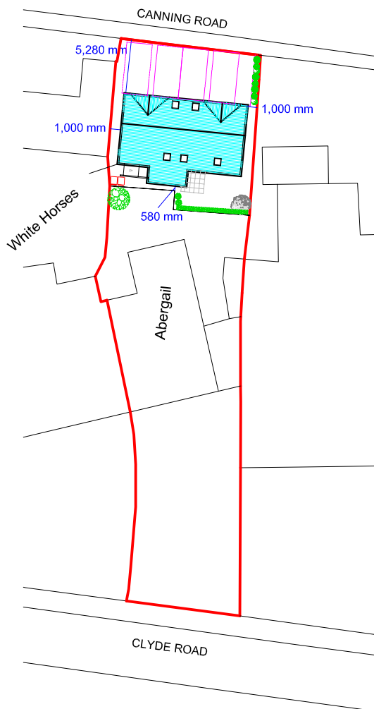
SITE PLAN - 1/500
