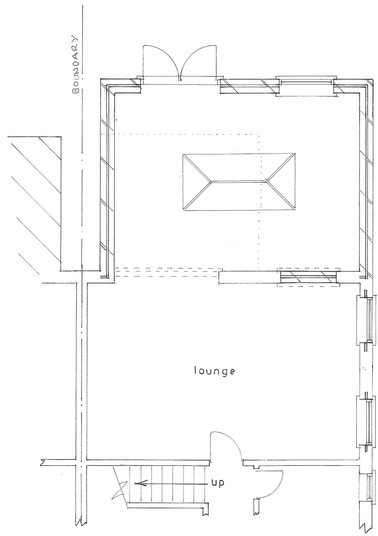
Plan 1 : 50
