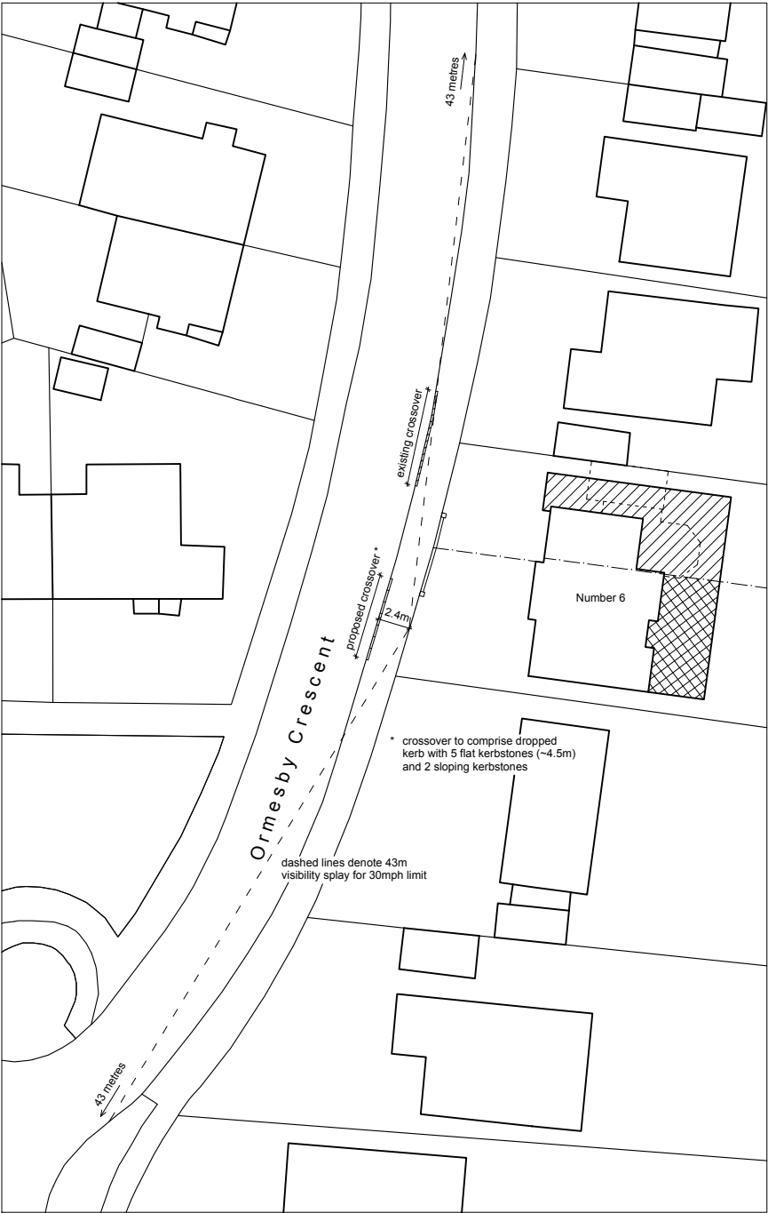
Crossover Plan Scale 1 : 500
