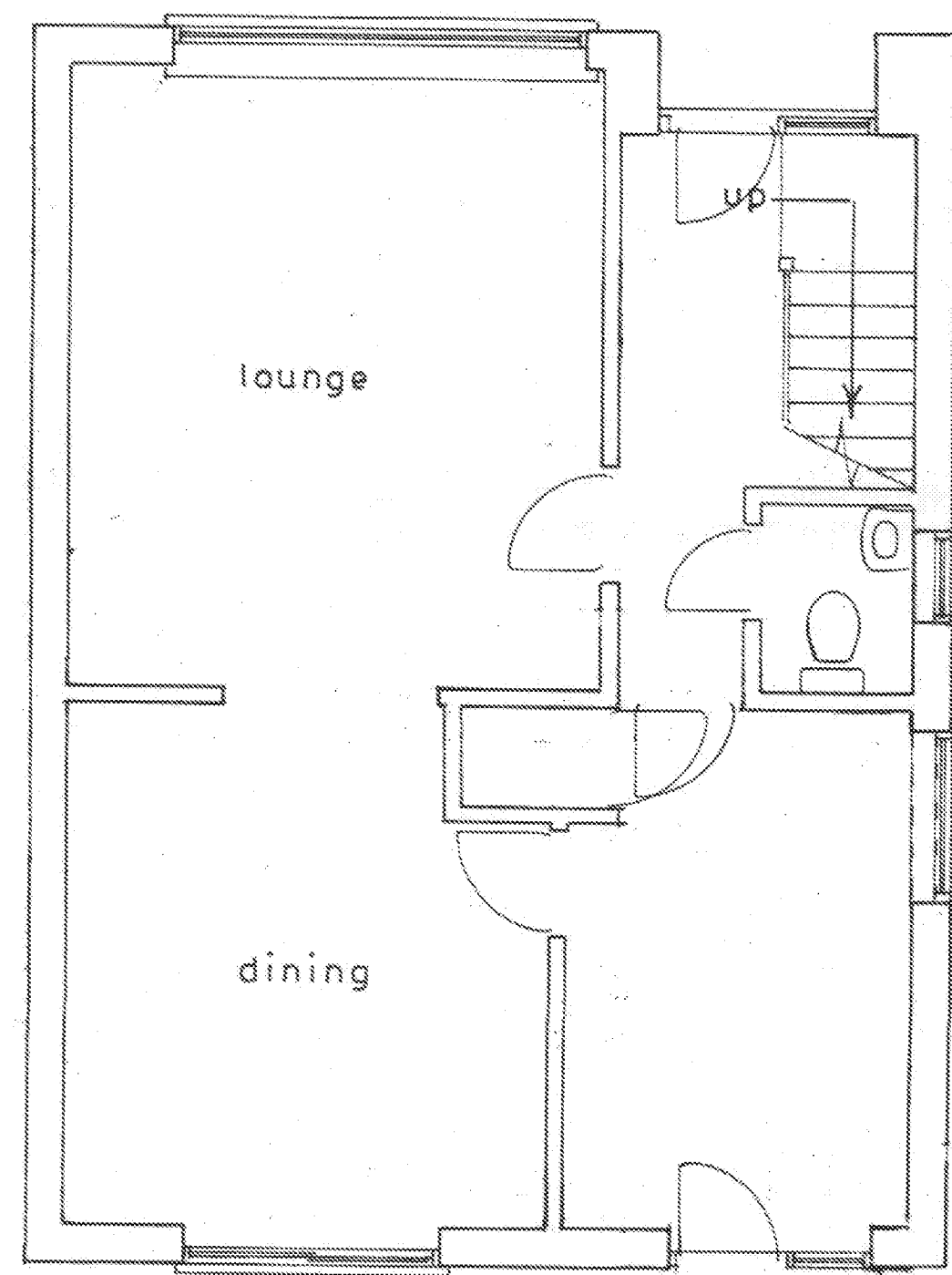
Plan 1 : 50
