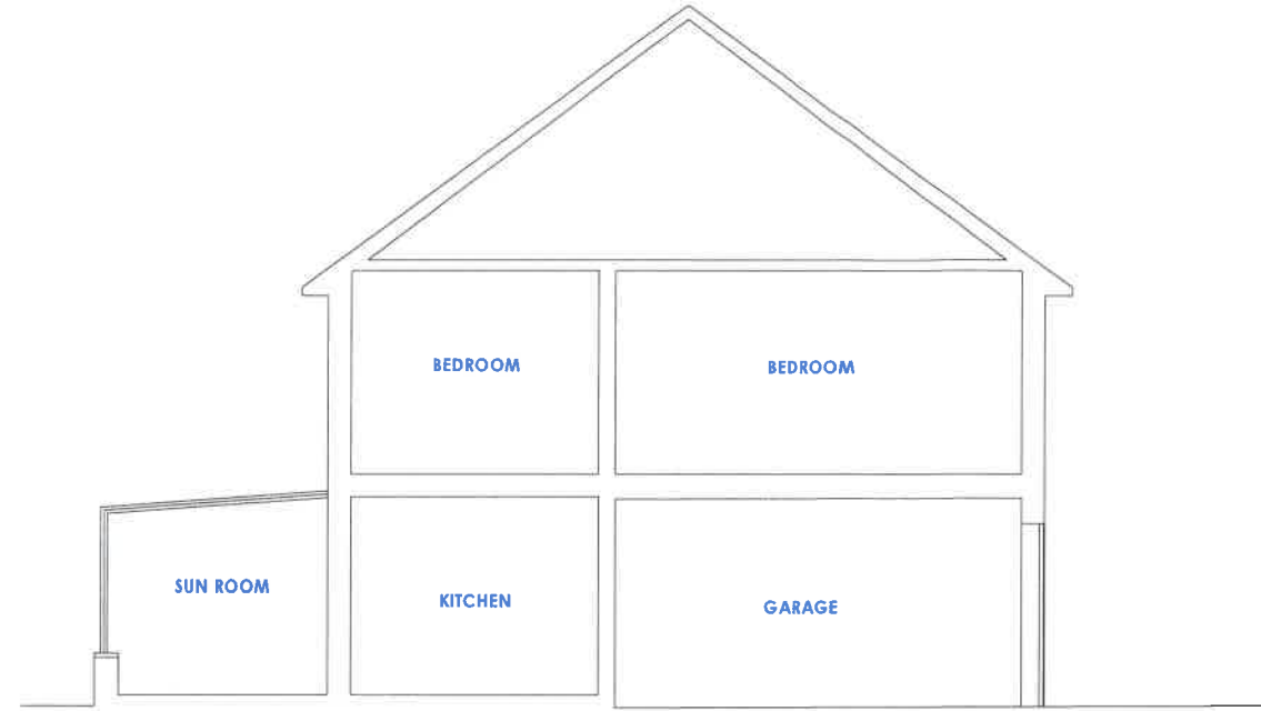
Section A-A
