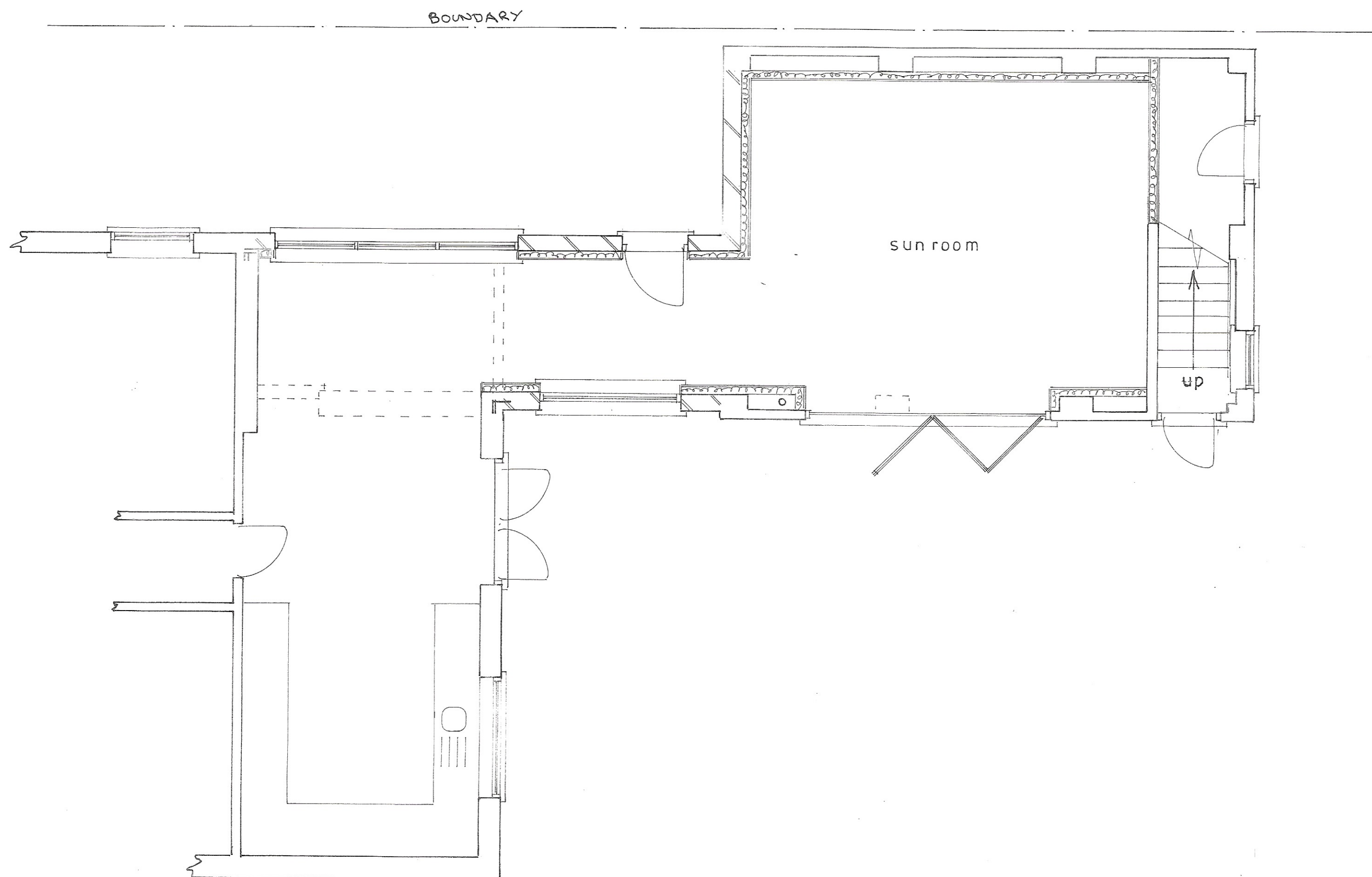
Plan 1 : 50
