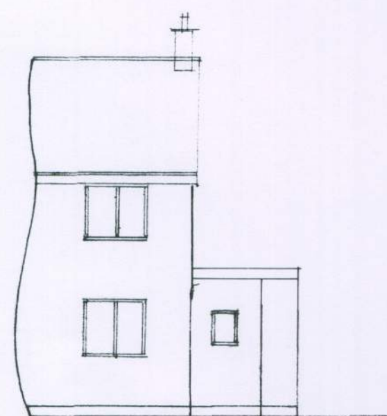
front 1 : 100
