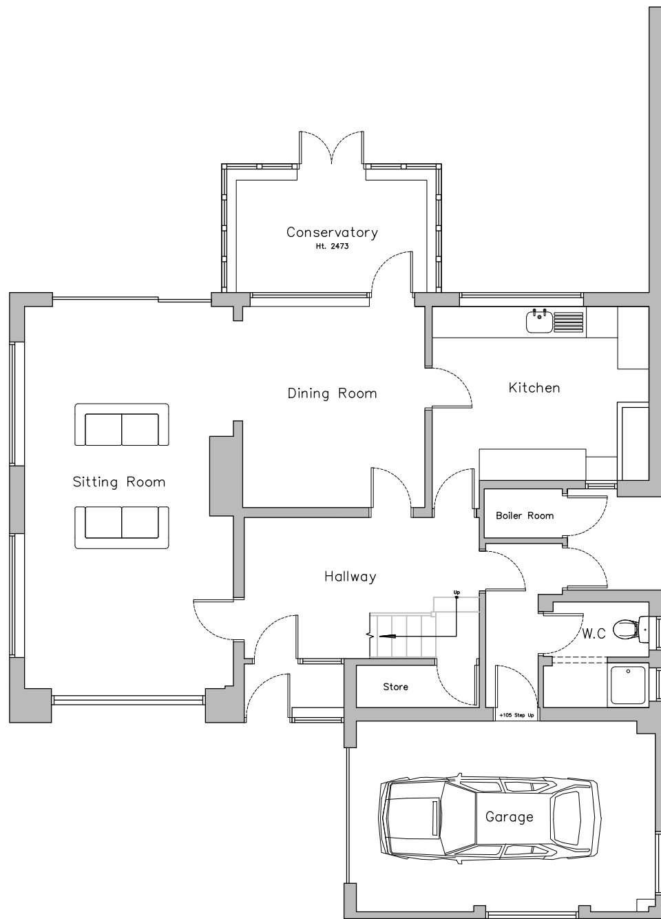
GF PLAN 1:100 @ A3
