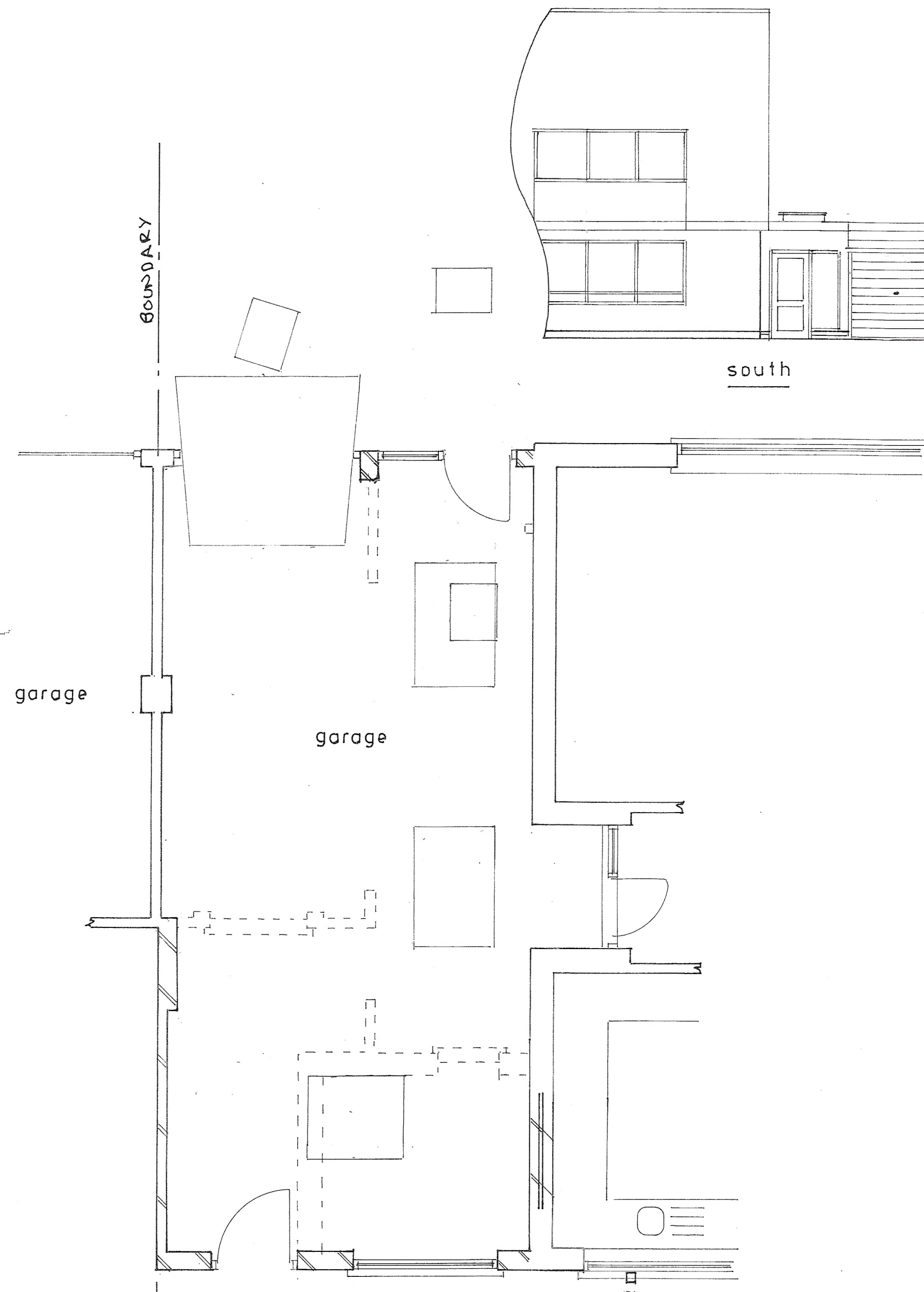
Plan 1 : 50
