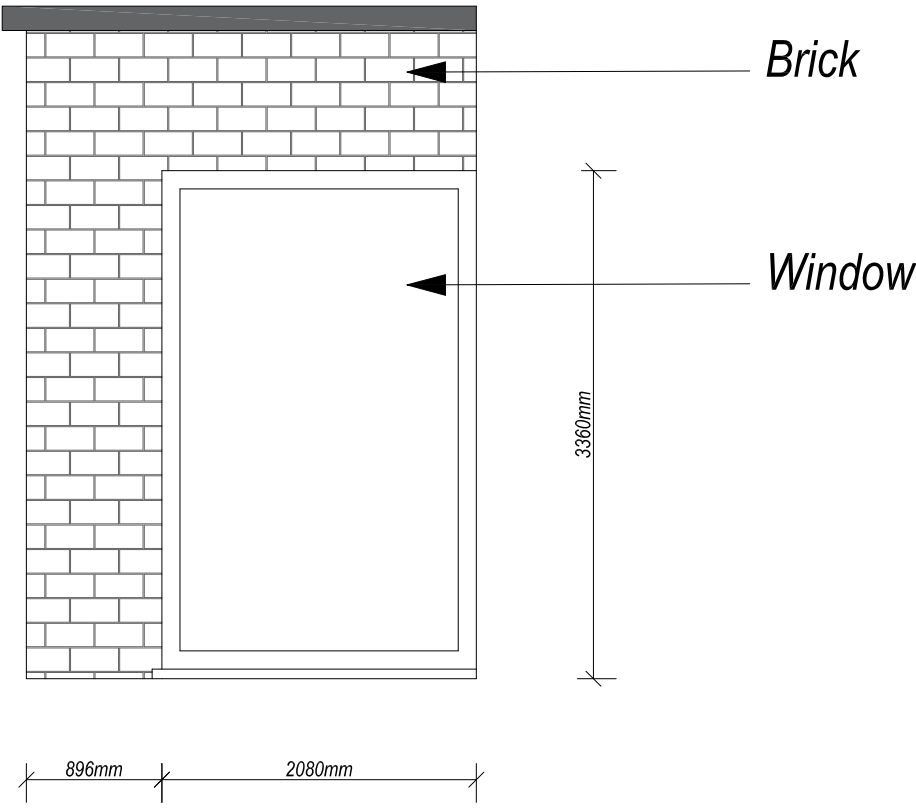
ELEVATION B
