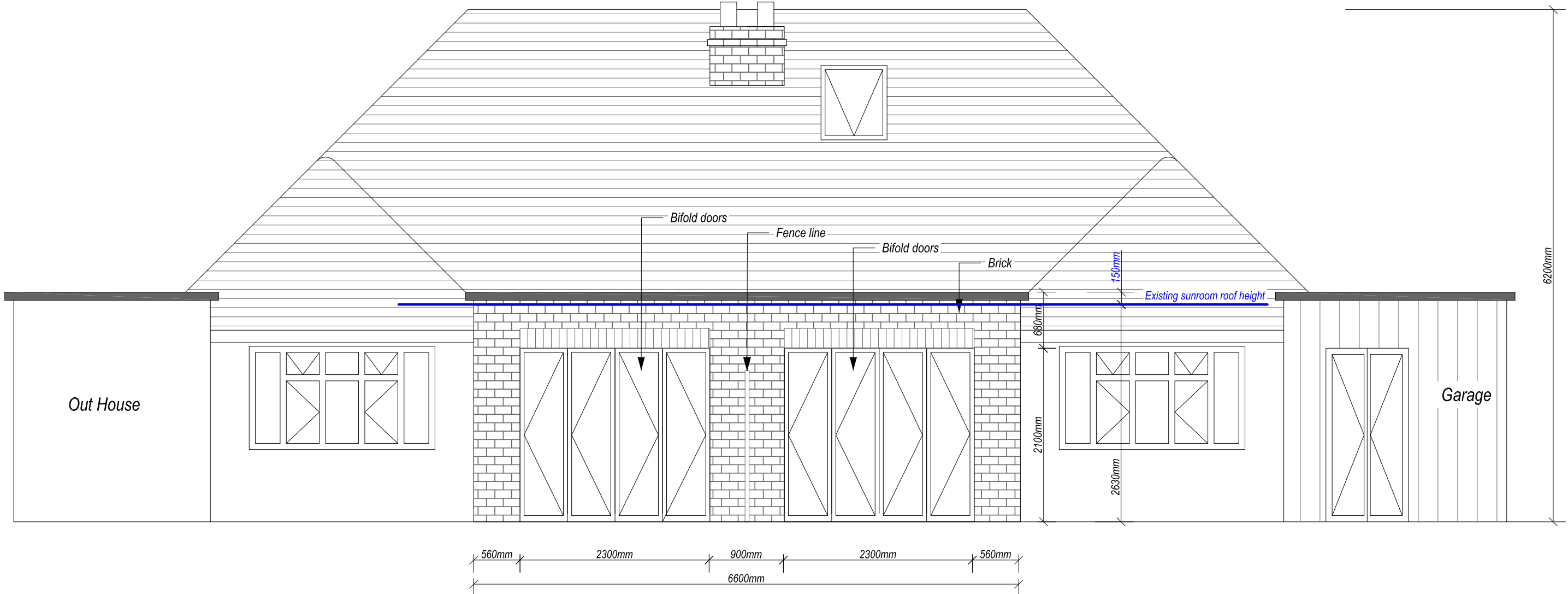
ELEVATION A
