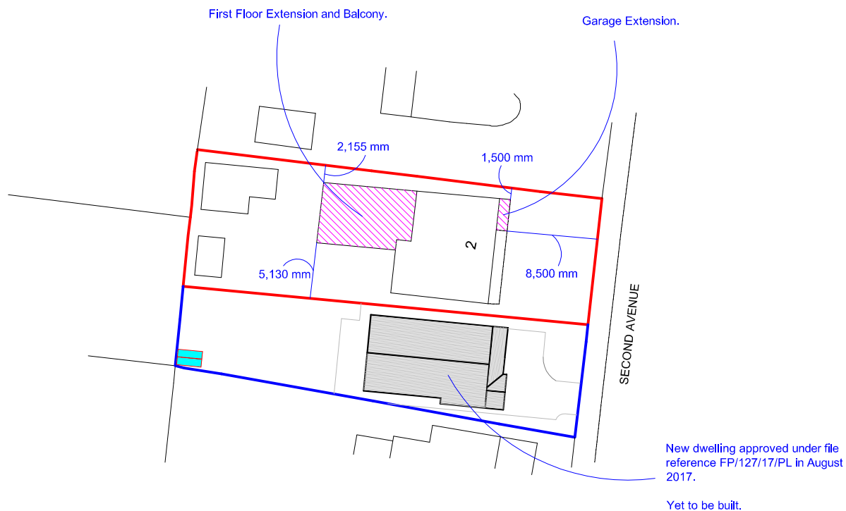
SITE PLAN - 1/500
