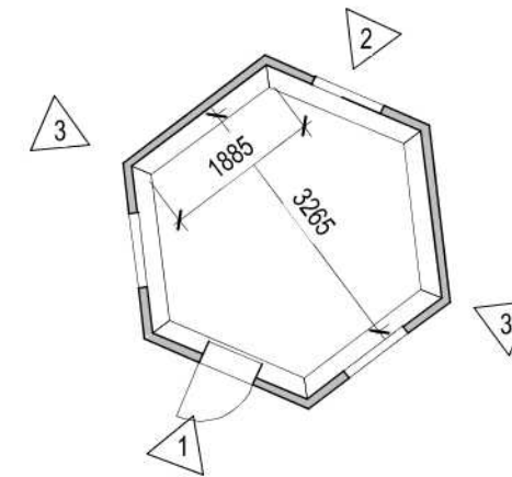
6 Cabin Layout 1 : 100
