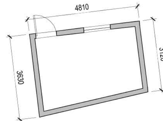
5 Shed - Plan 1 : 100
