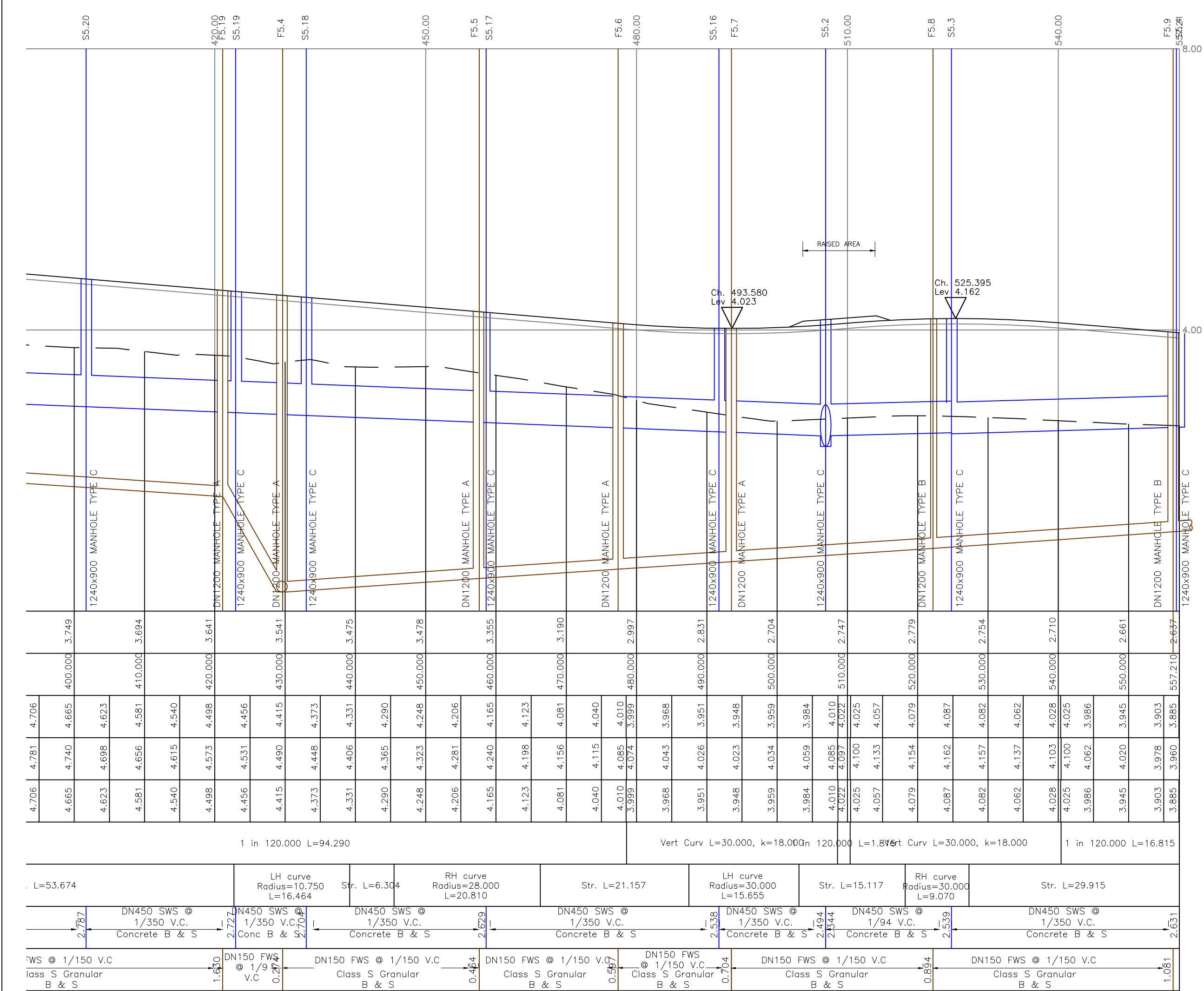
Road 24 Horiz. 1:500 Vert. 1:50
