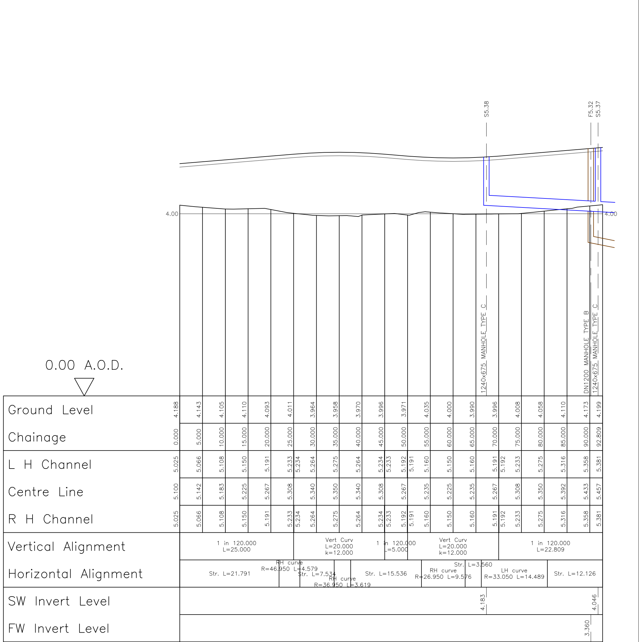
Access 4 Horiz. 1:500 Vert. 1:50
