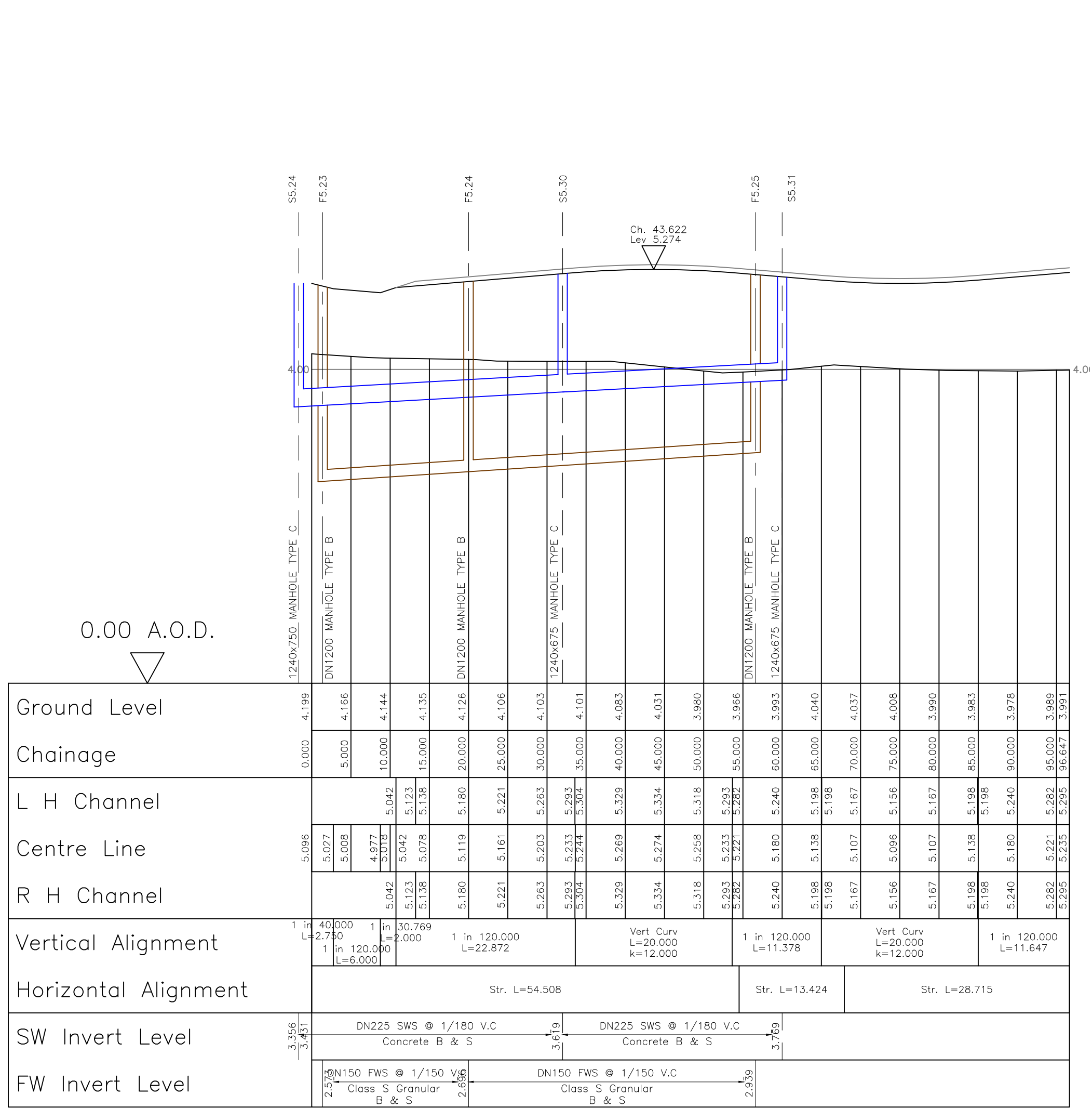
Access 2 Horiz. 1:500 Vert. 1:50
