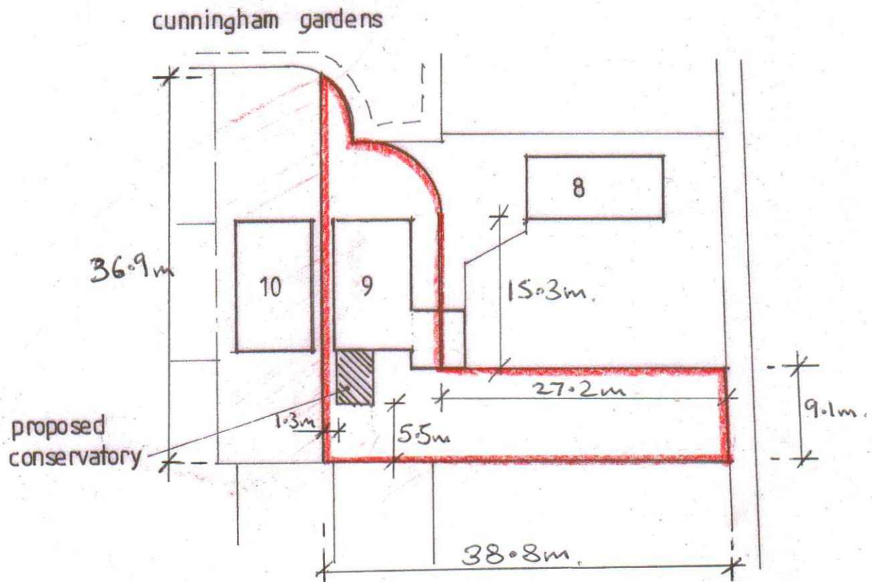
SITE PLAN 1:500
