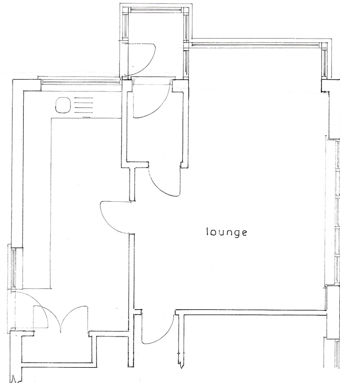
Plan 1 : 50
