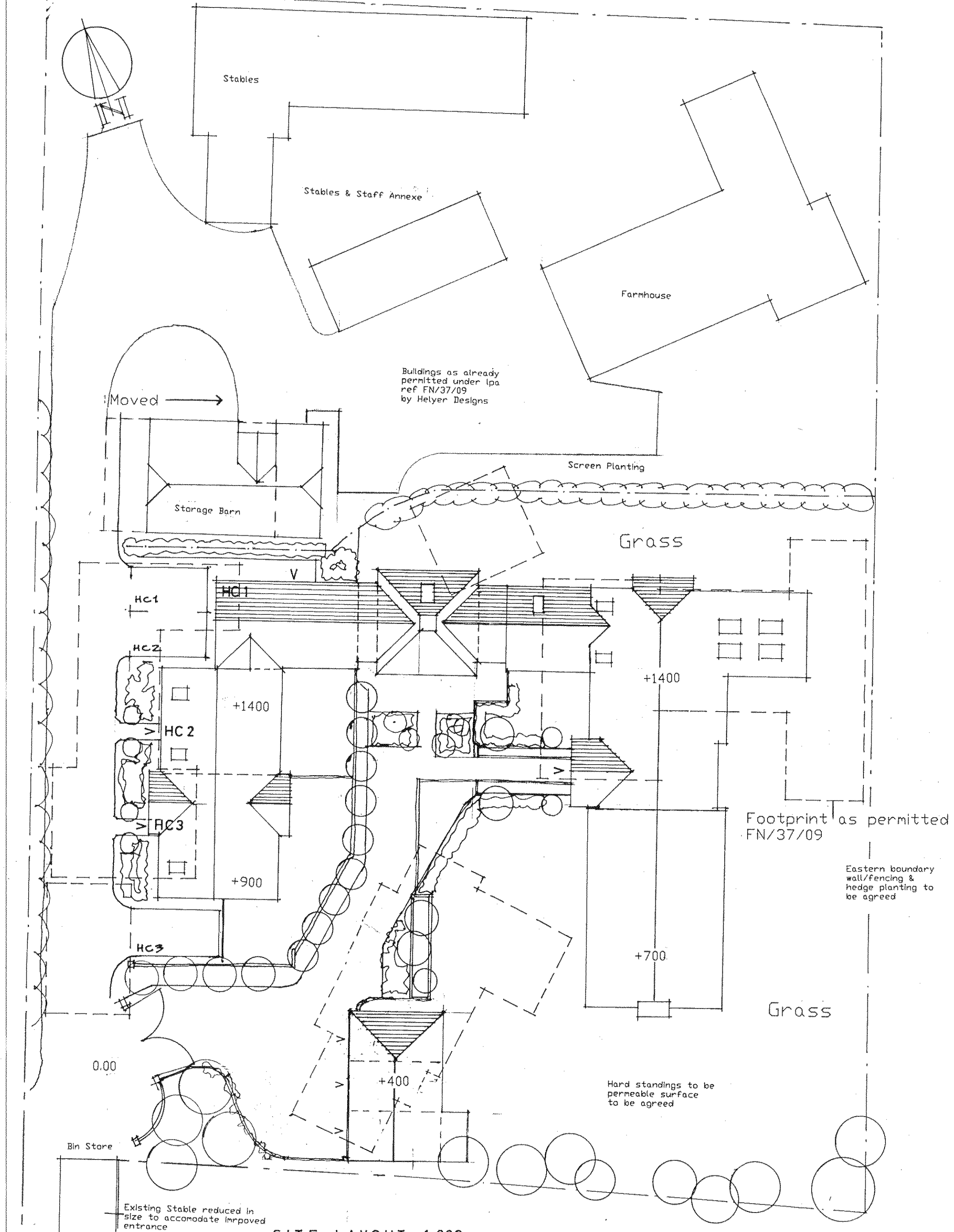
SITE LAYOUT 1:200
