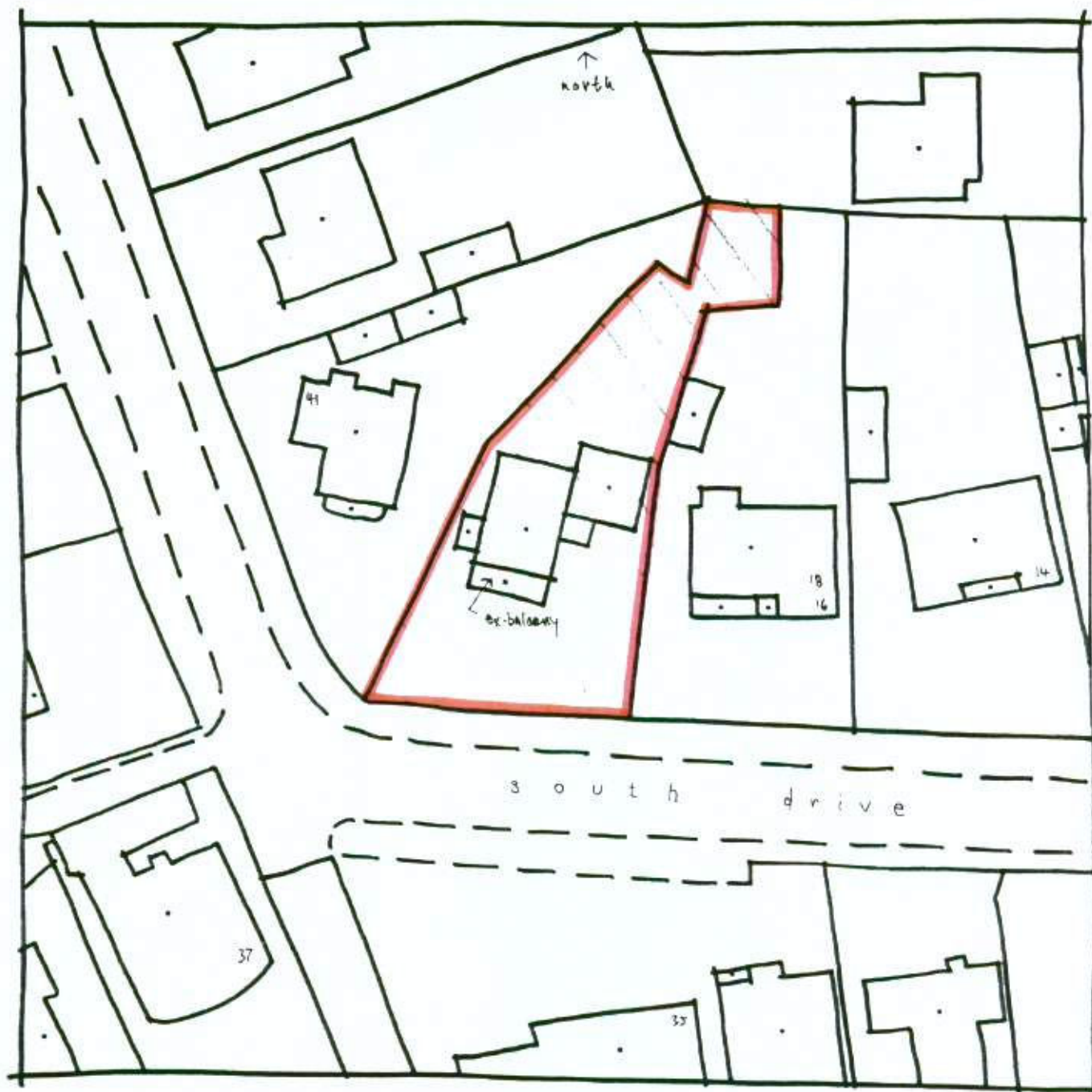
SITE PLAN 1:500
