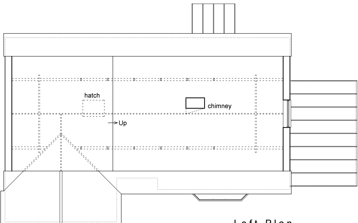
Loft Plan
