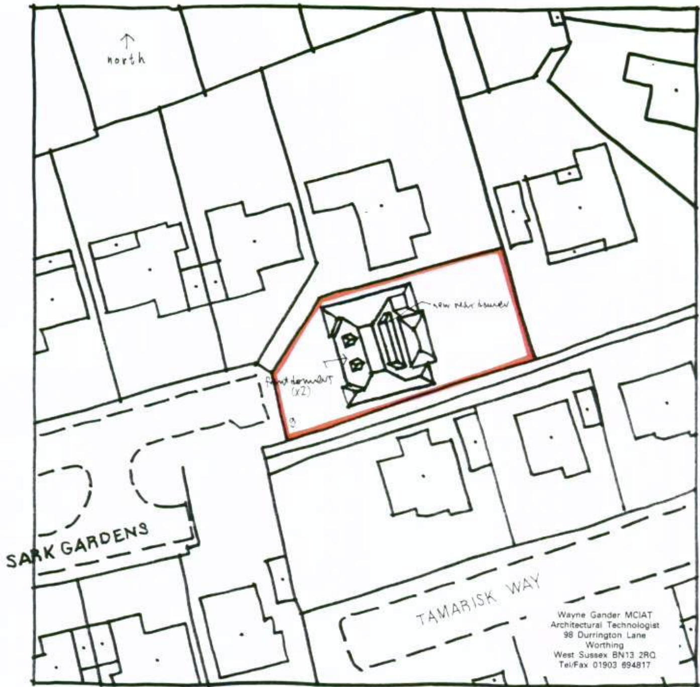
SITE PLAN 1:500
