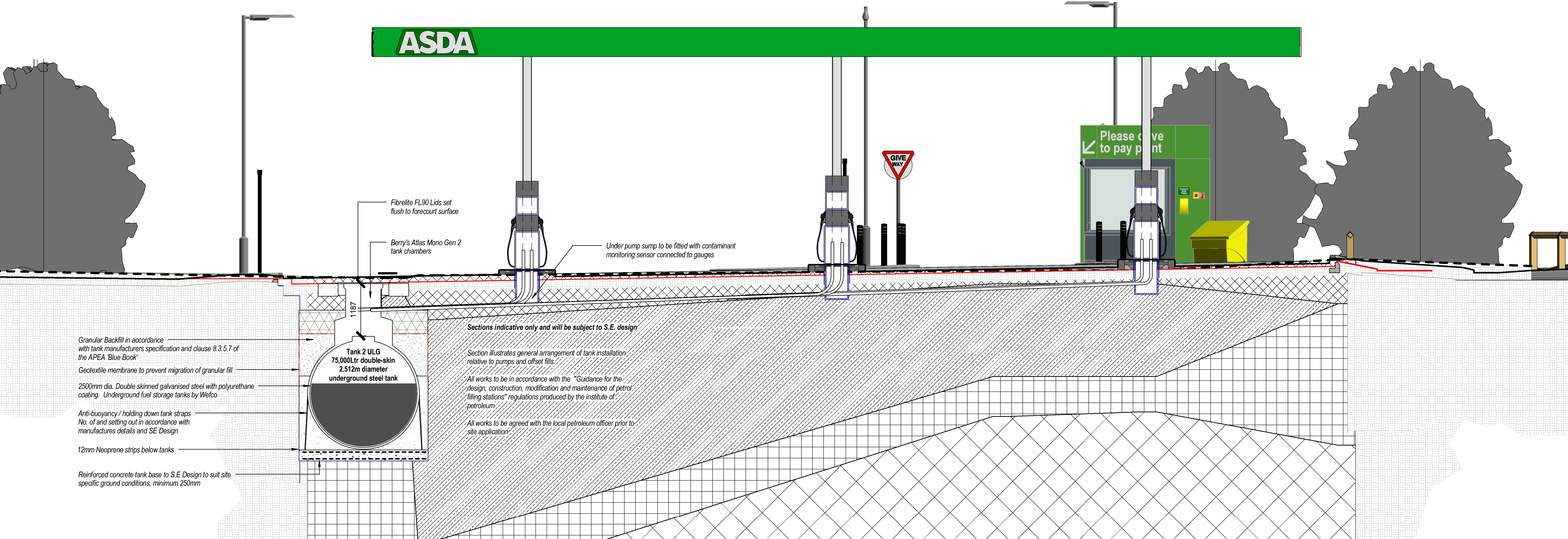
Forecourt Longitudinal Section Copy 1 1 : 50
