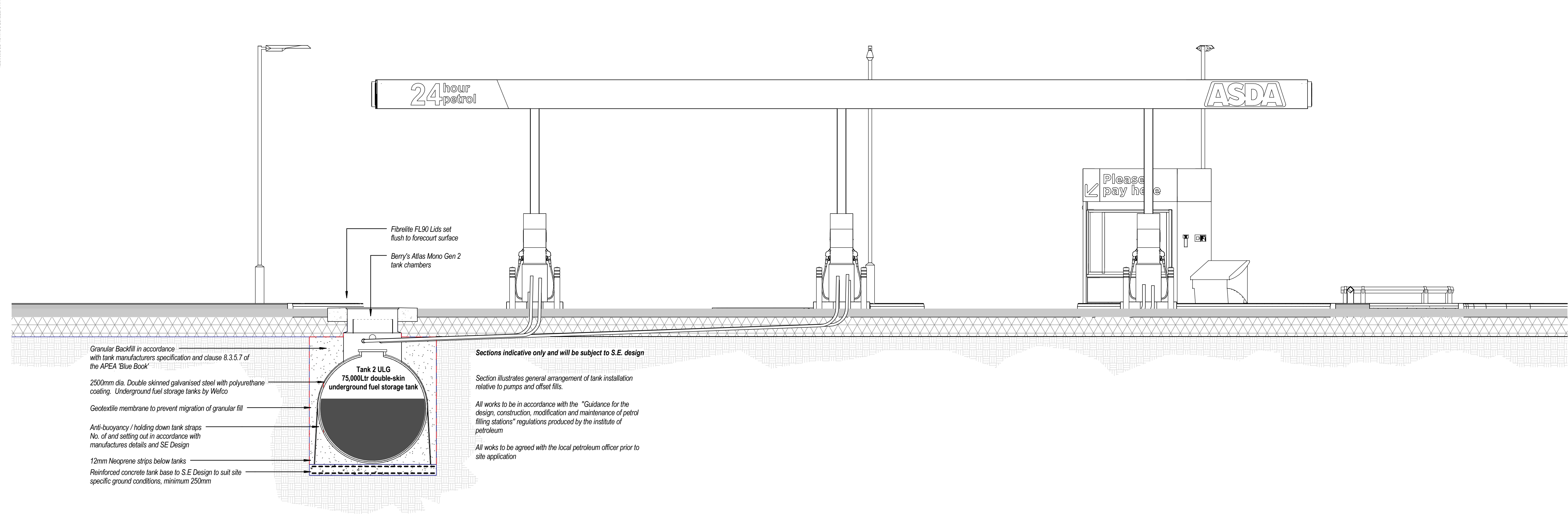
Forecourt Longitudinal Section 1 : 50
