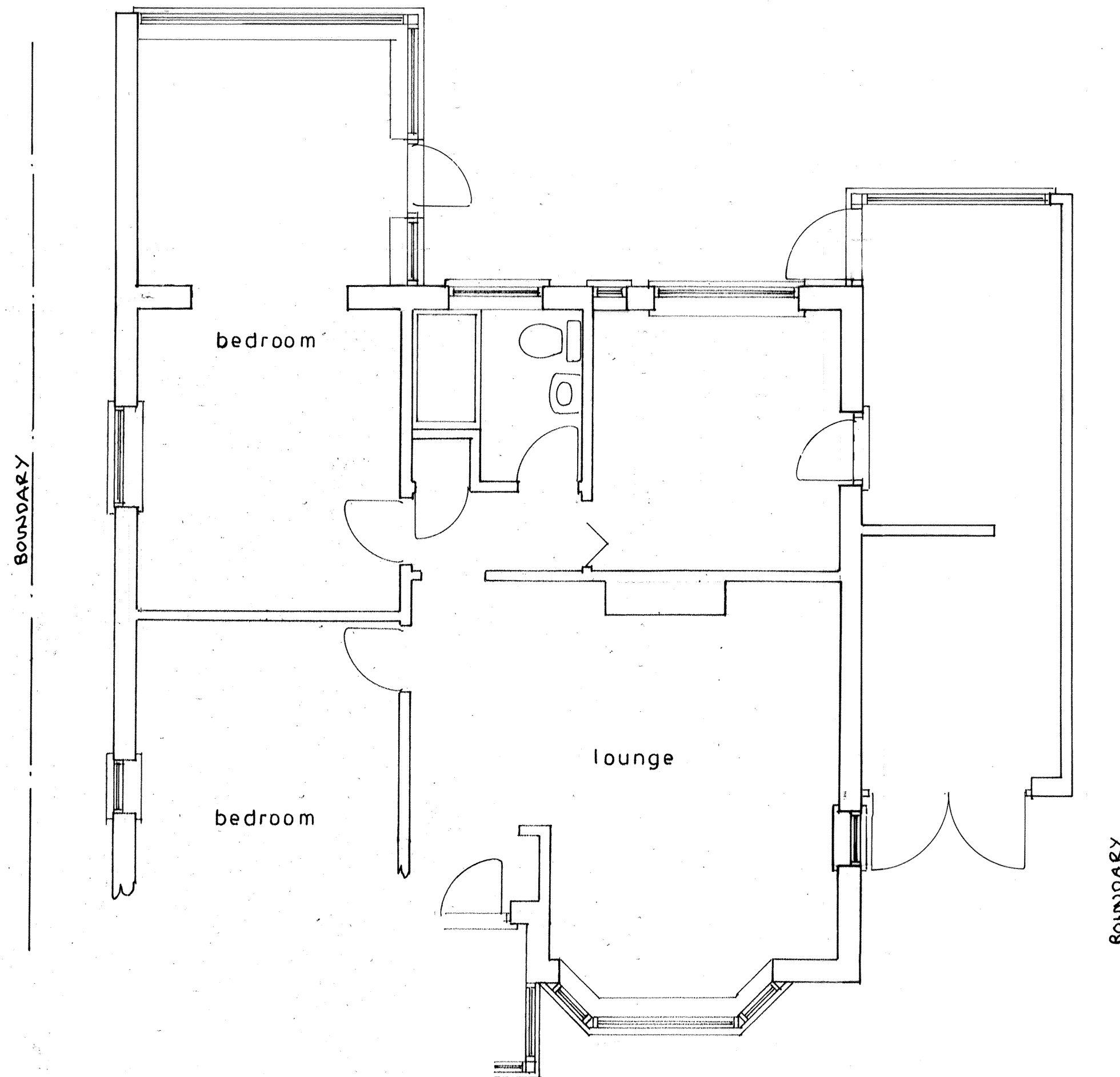
Plan 1 : 50 Existing
