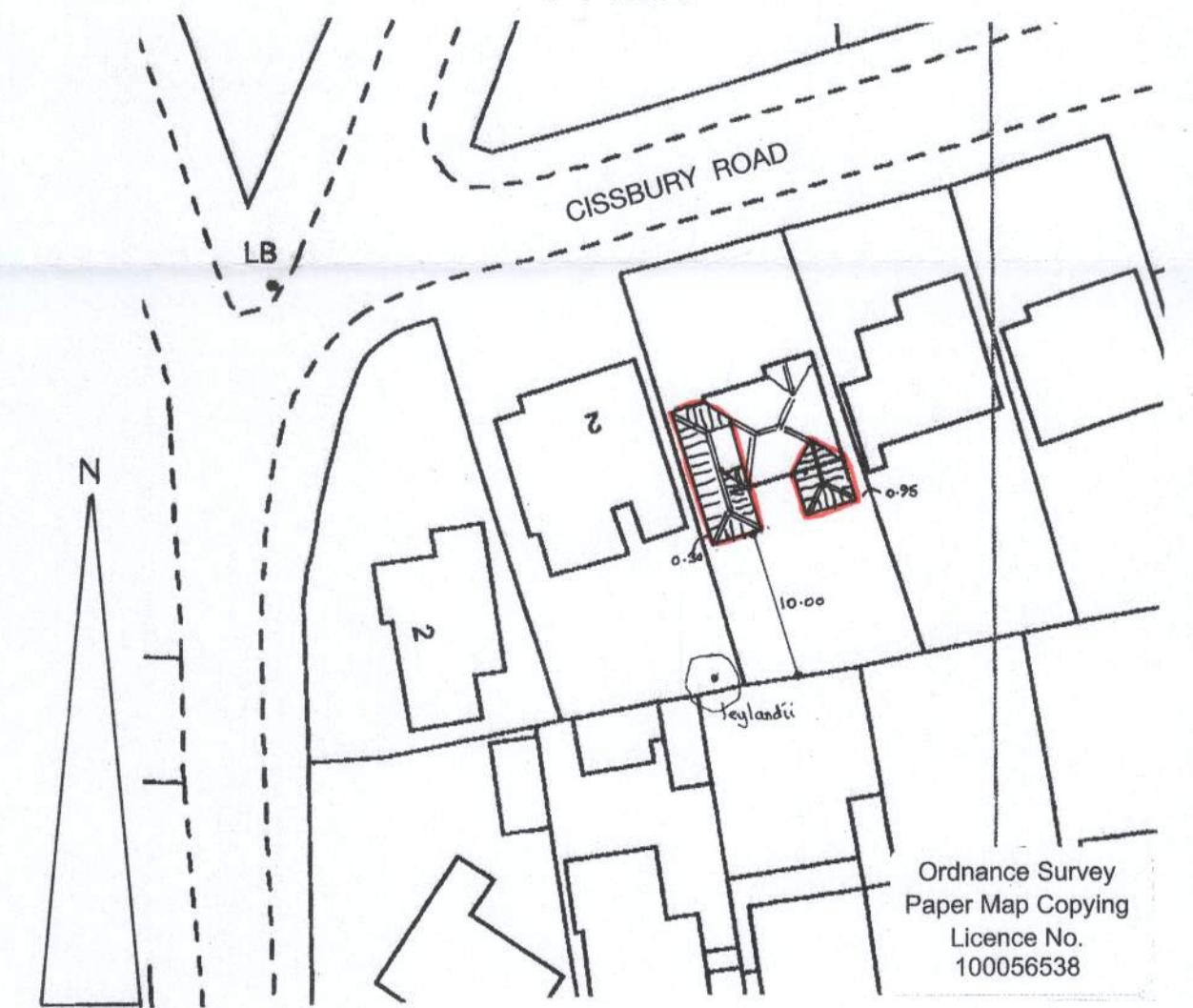
block plan 1 : 500
