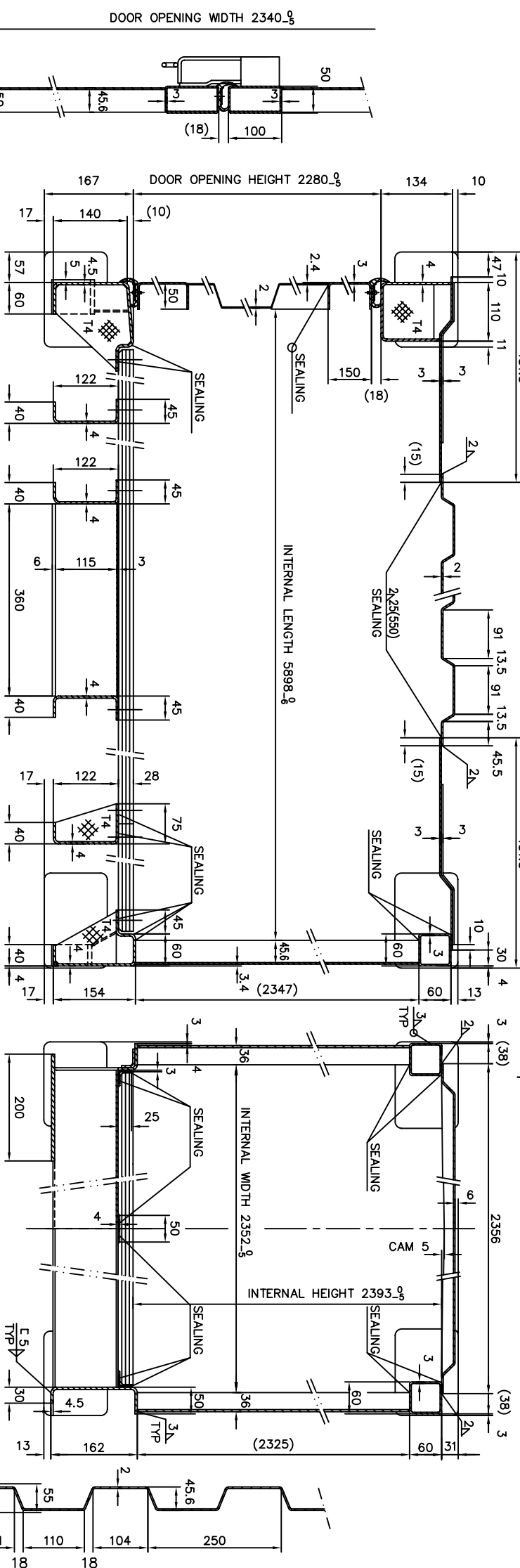
SECTION D-D
