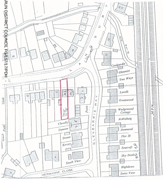
Site plan 1:1250
