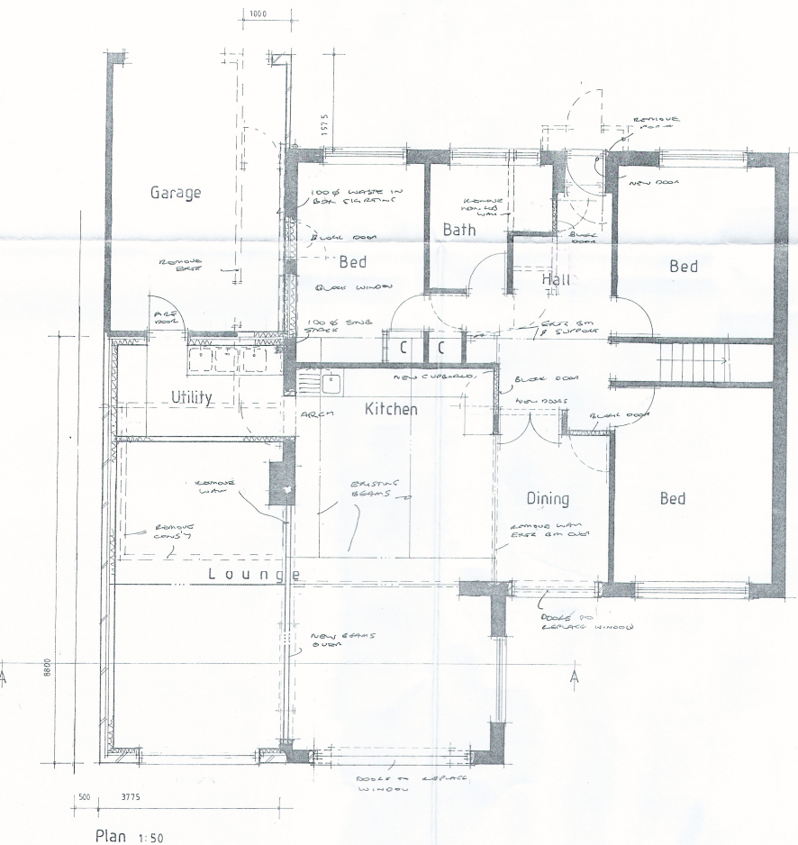
Plan 1:50
