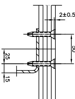
SECTION E-H 1 : 2
