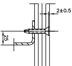
SECTION E-H 1 : 2
