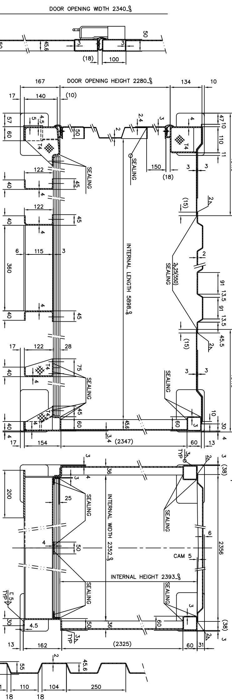
SECTION A-A 1 : 5
