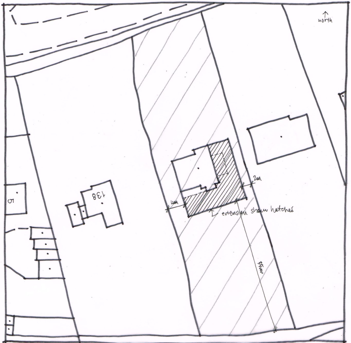
SITE PLAN 1:500
