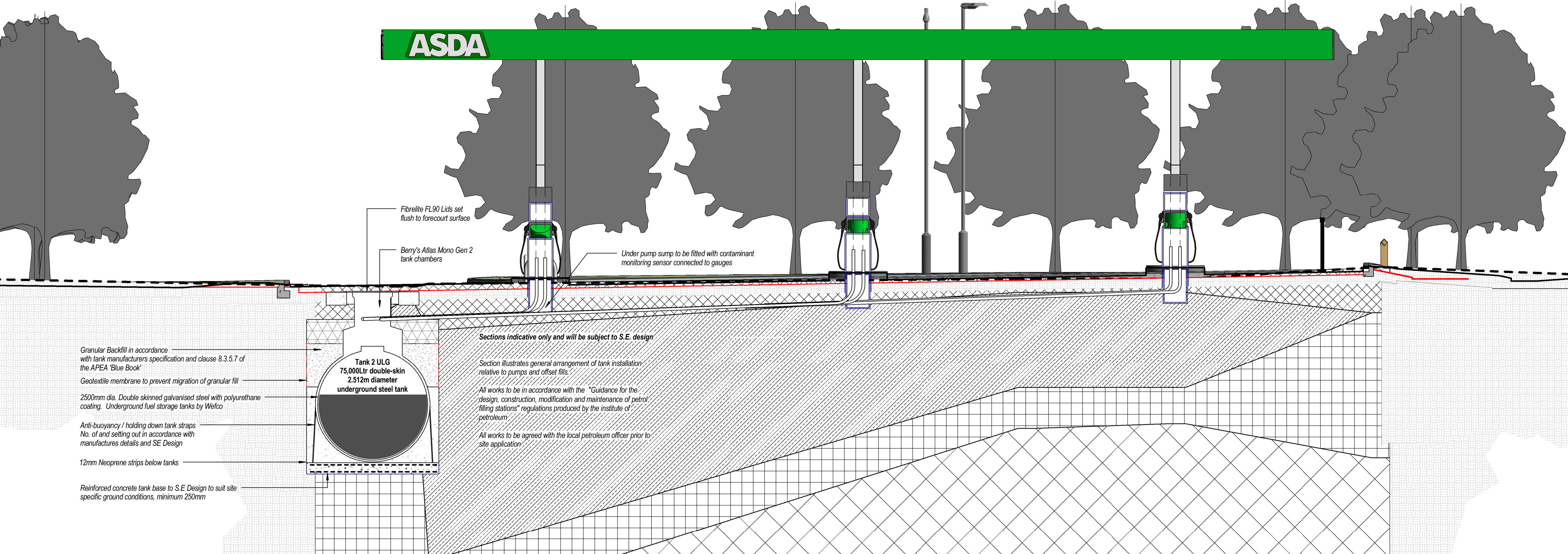
Forecourt Longitudinal Section Copy 1
