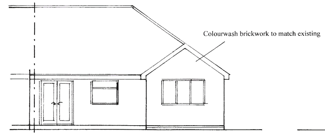
north 1 : 100
