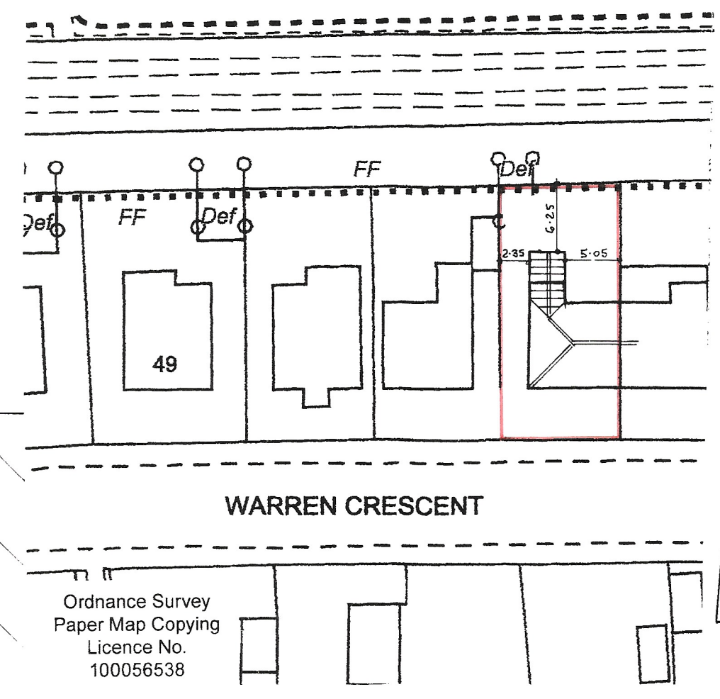
block plan 1 : 500
