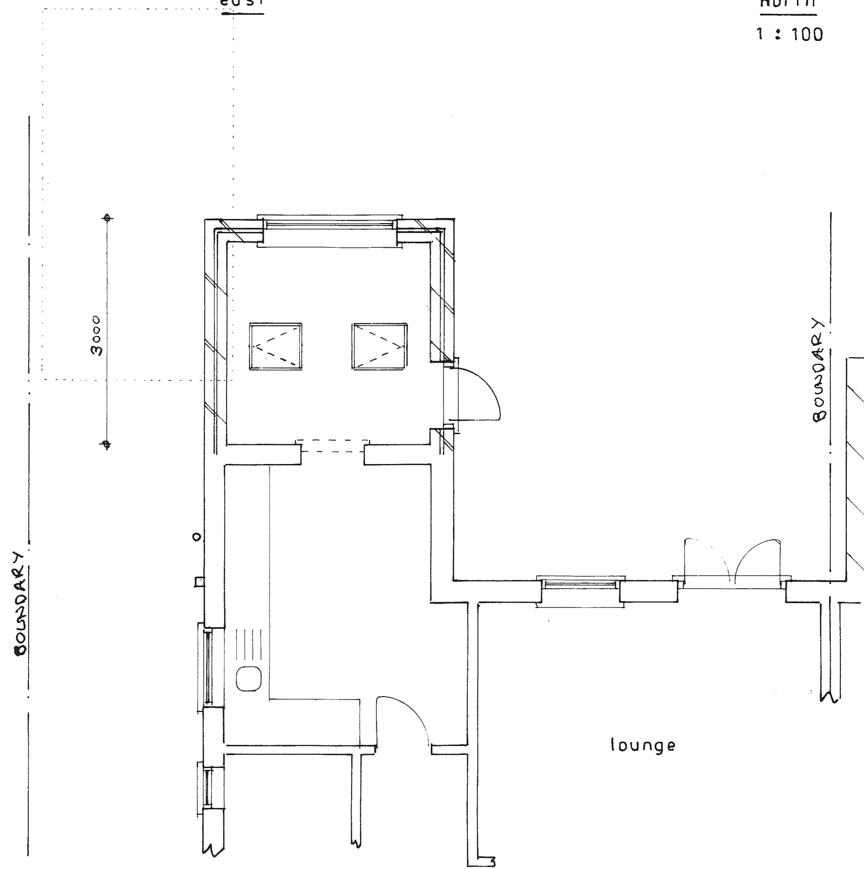
Plan 1 : 50
