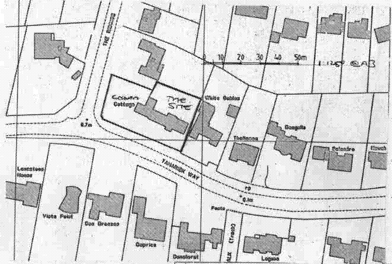
Site plan 1:1250
