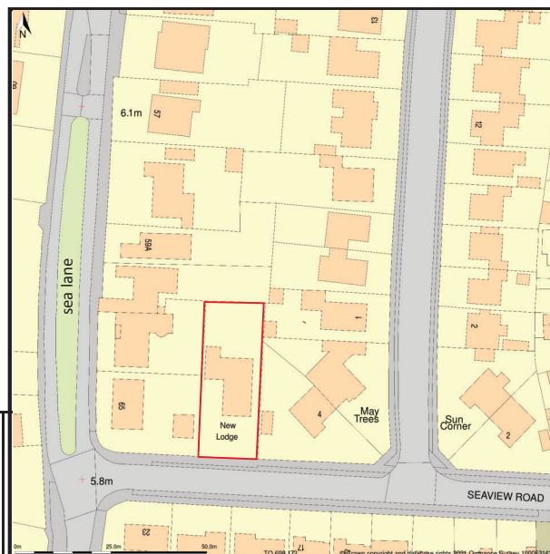
SITE PLAN 1:1250
