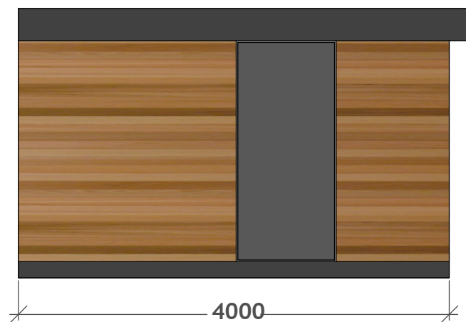
LEFT SIDE
