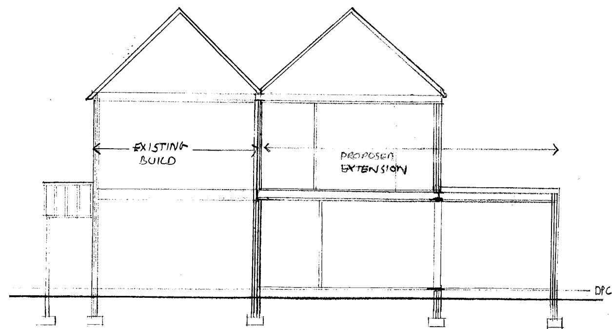
SECTION A-A 1:100
