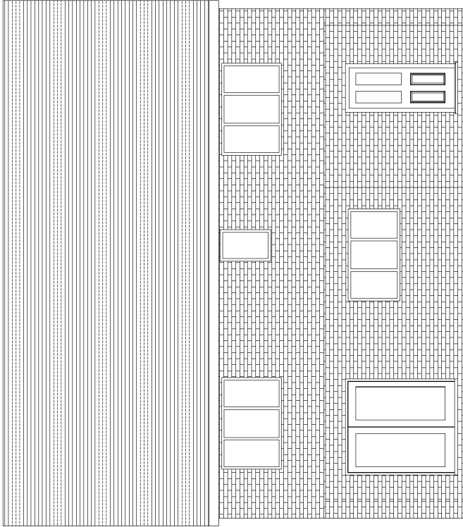
Existing SE Elevation 1 : 100
